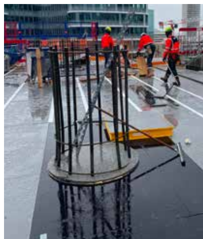
Alphi peut dimensionner et fabriquer des éléments spéciaux pour répondre aux besoins spécifiques du chantier. Ici : un coffrage poteau
